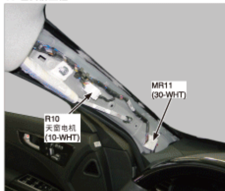
55.左侧前立柱
